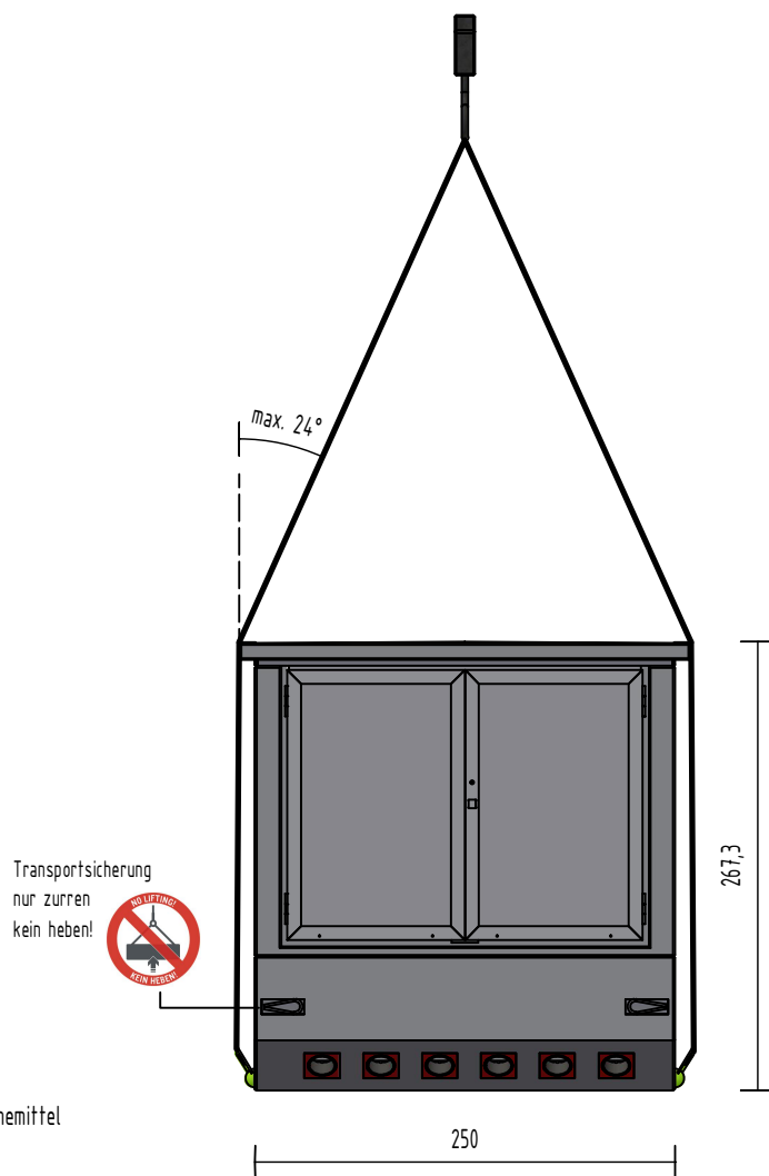
Station Stirnseite
