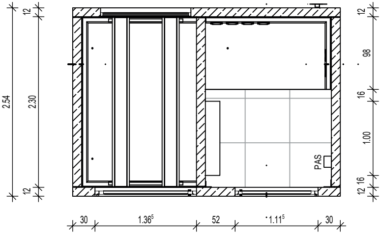
Grundriss
